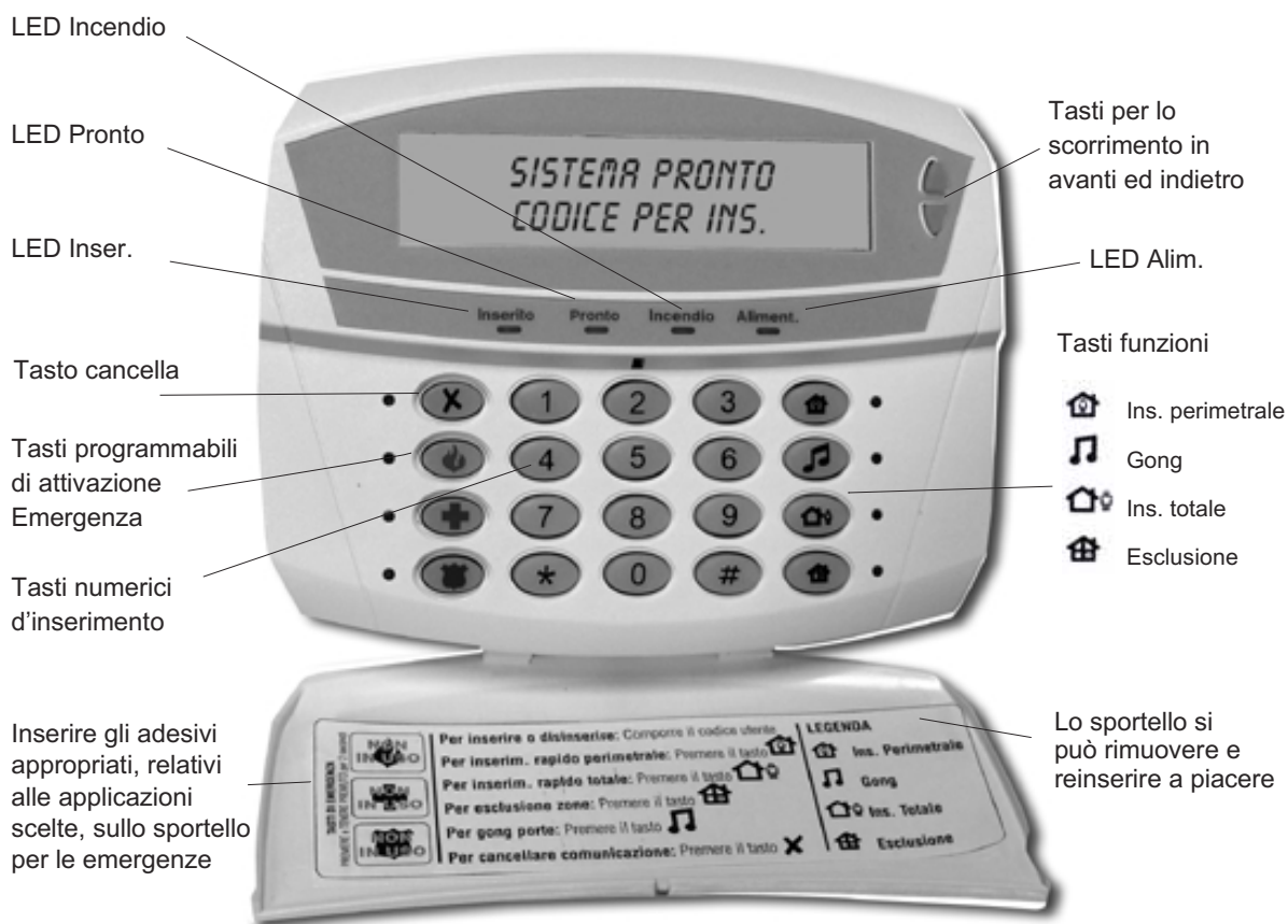
La tastiera LCD NX-1192
