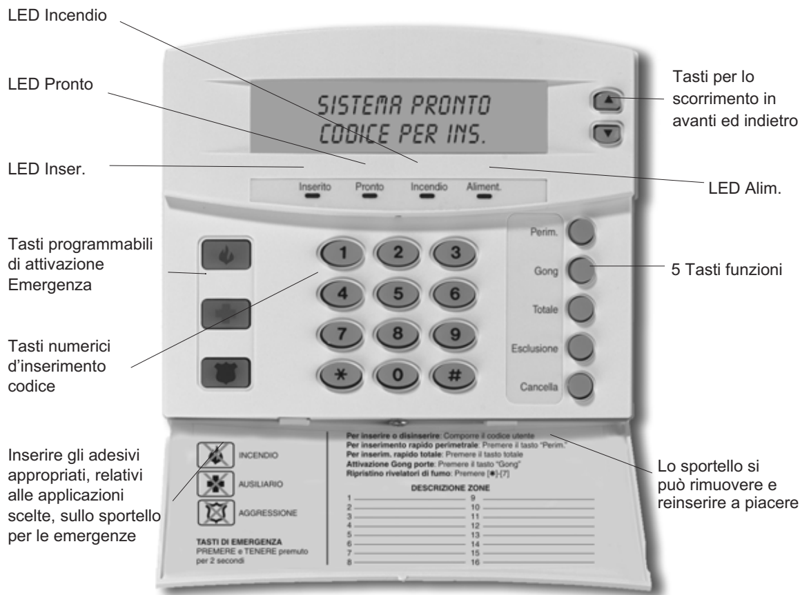
La tastiera LCD NX-148
